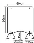
507CR Mampara protectora de acrílico Peso: 1.4kg
