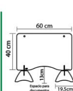
506CR Mampara protectora de acrílico Peso: 1.0kg
